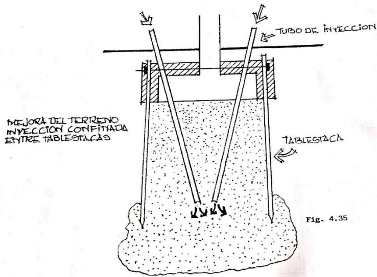
Figura 33 Cimentaciones contemporáneas
