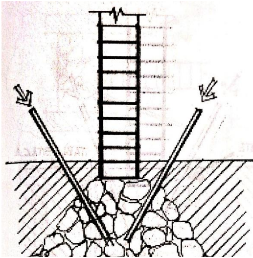
Figura 32 cimentaciones antiguas
